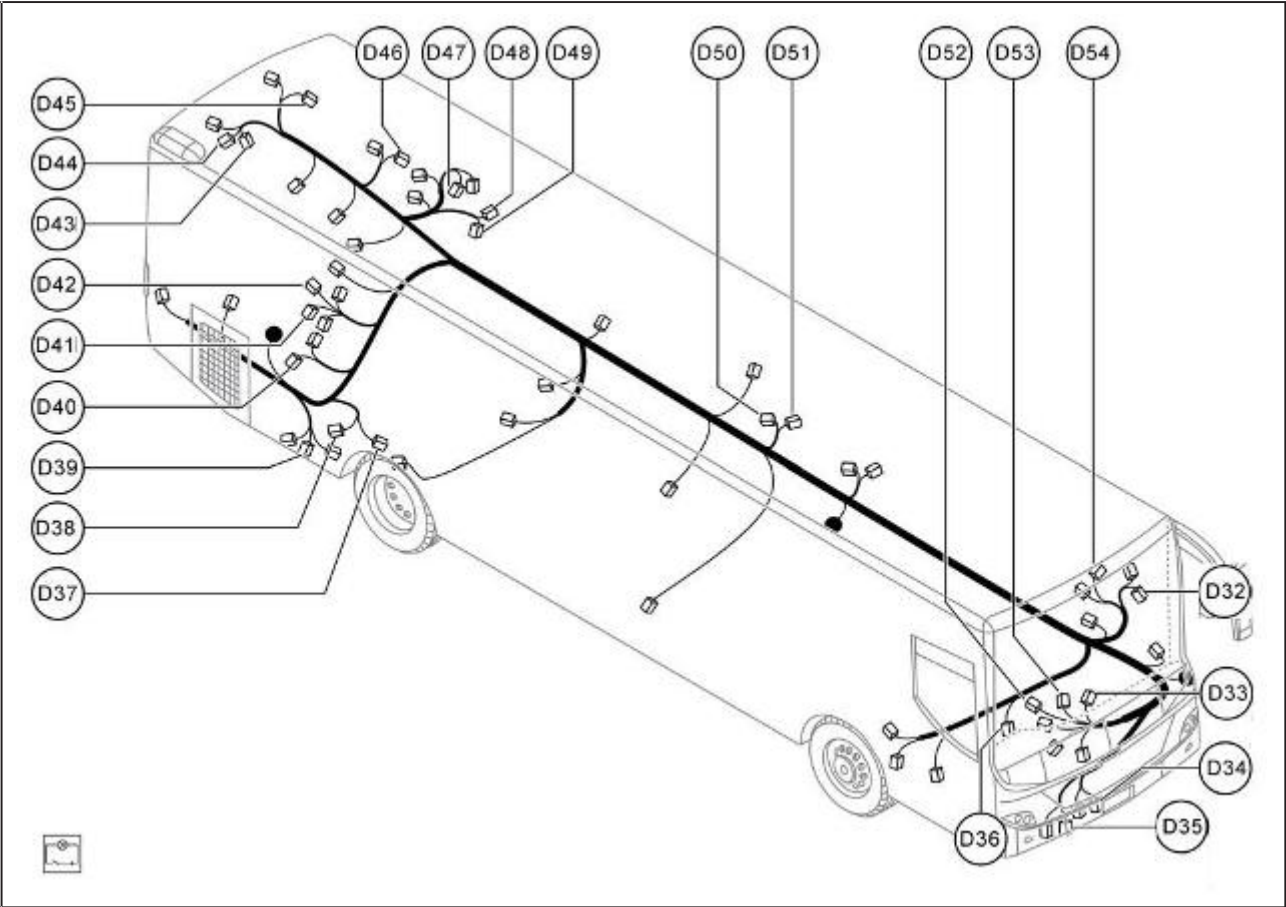
底盘线束连接示意图二
