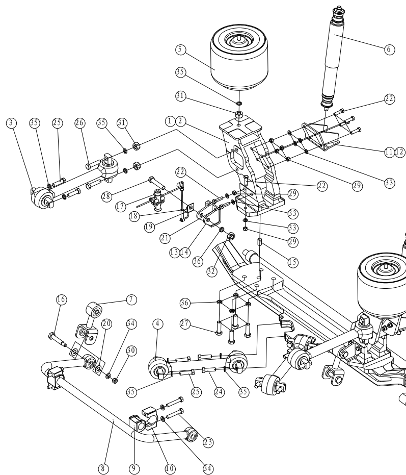
DWG11F 前悬结构示意图:
