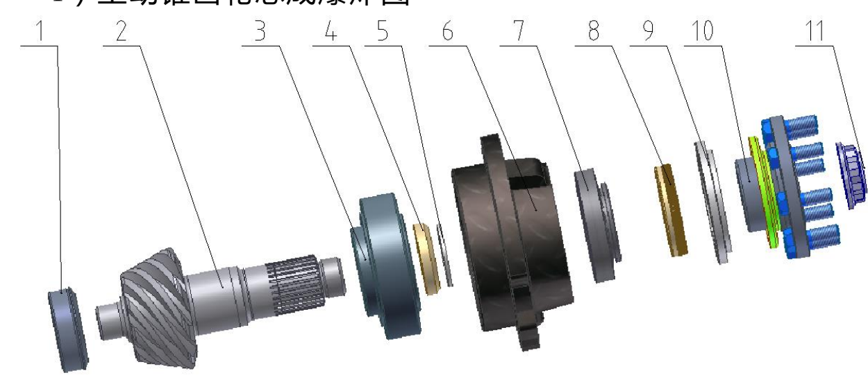
图 2-5：主动锥齿轮总成轴测分解图
