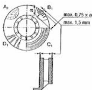
图 4-12: 表面裂纹检查
