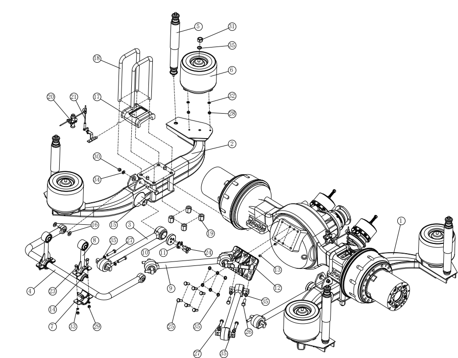
DWG13R 后悬结构示意图:
