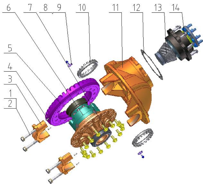
1) 主减速器总成爆炸图
