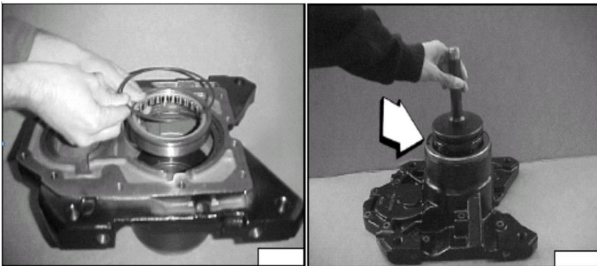
装缓速器后支架
