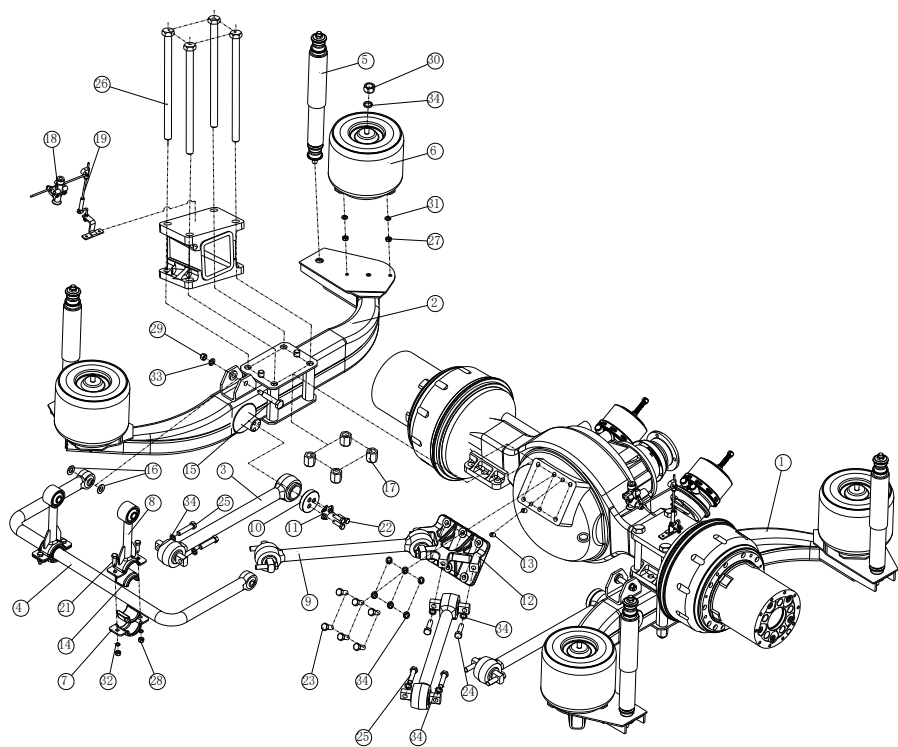
DW11F 前悬结构示意图:
