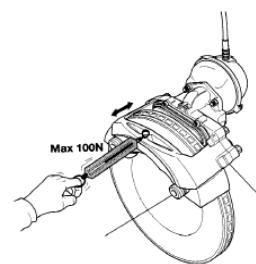
图 4-14 滑销间隙检查
